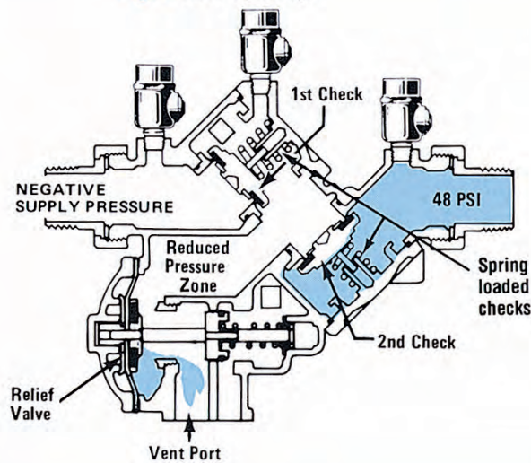
Fig. 3 Back Siphonage
