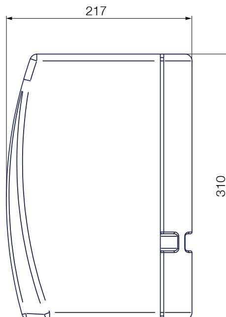
Isolierschale FlowBox DN 20
