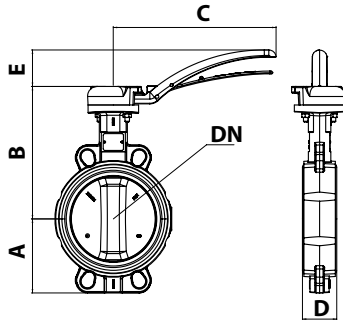
Sylax und Sylax Gas Hebel aus Gusseisen, Zwischenflansch Scheibe: Gusseisen/Edelstahl 316/ Aluminiumbronze
