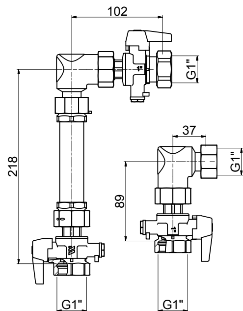
WMZ2029-V2-Ni
