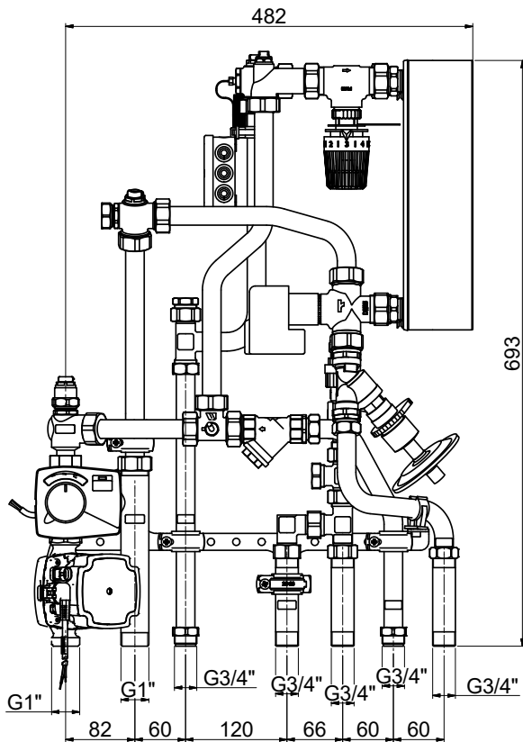
HIU2 HKM
