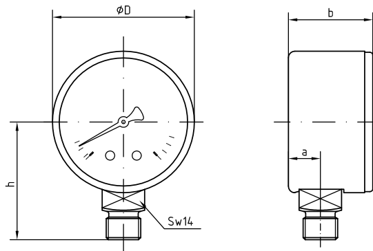
F+R 250
