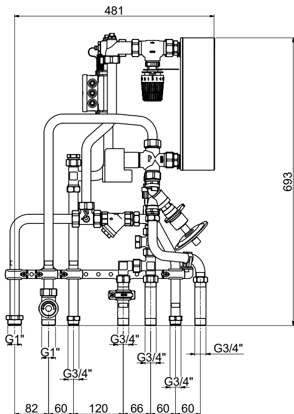
HIU2 HK
