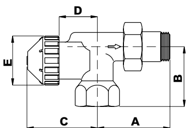
TVE-S
