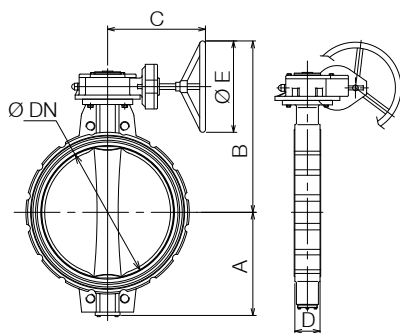
Sylax mit Handgetriebe ZWISCHENFLANSCH Scheibe: Gusseisen/Edelstahl 316
