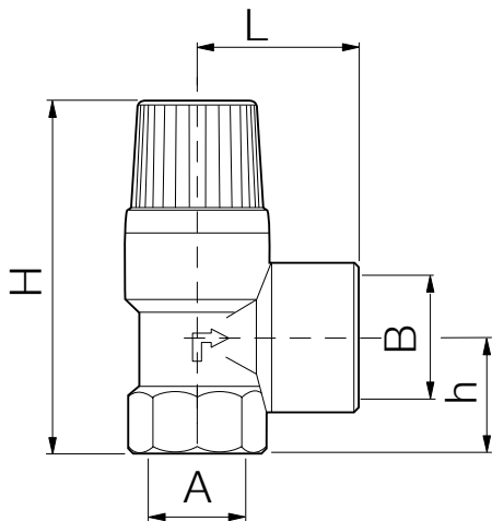
SVH
