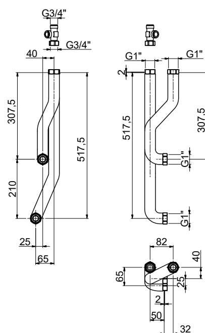
ANSCHLUSSET HKM-HT
