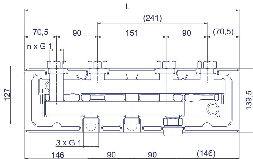
VB20
