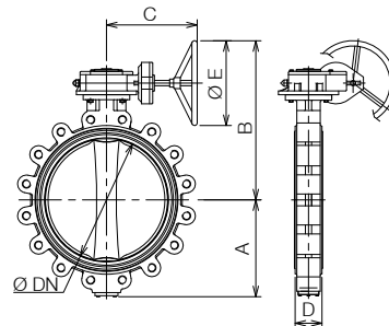
Sylax mit Handgetriebe ENDFLANSCH Scheibe: Gusseisen/Edelstahl 316
