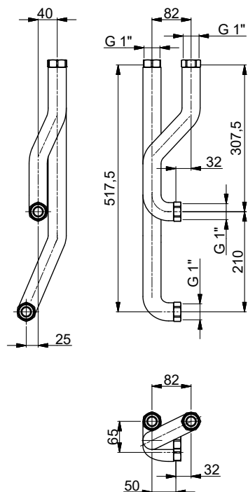
ANSCHLUSSET HKM
