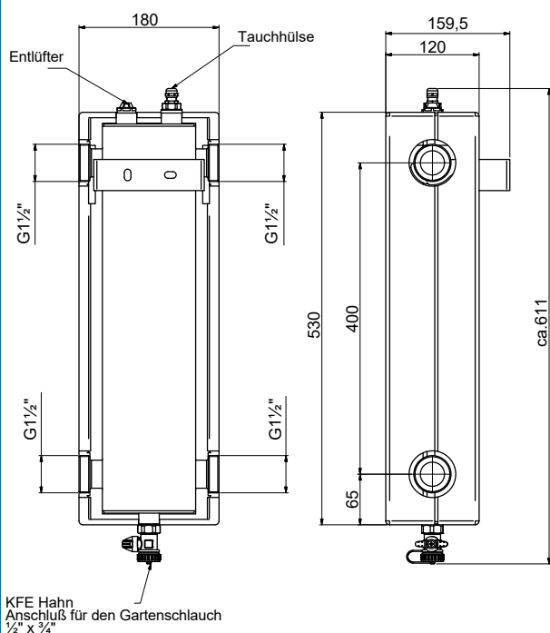
HW 80/120, 4 m³/h
