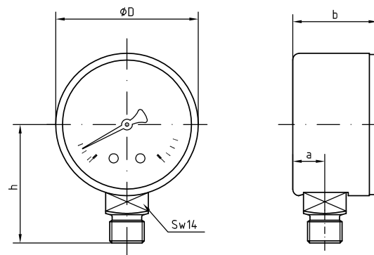
F+R 200, F+R 201
