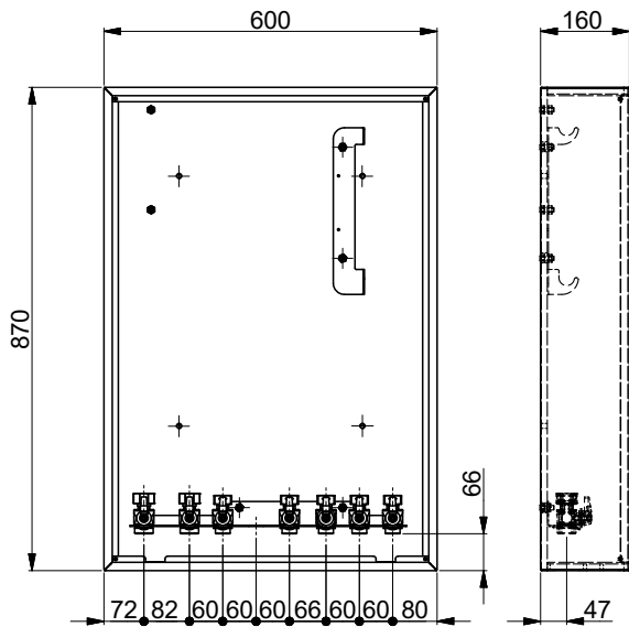
HIU2AI
