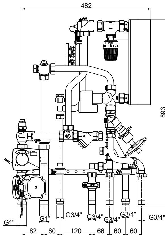
HIU2 HKM
