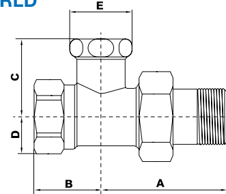
RLD
