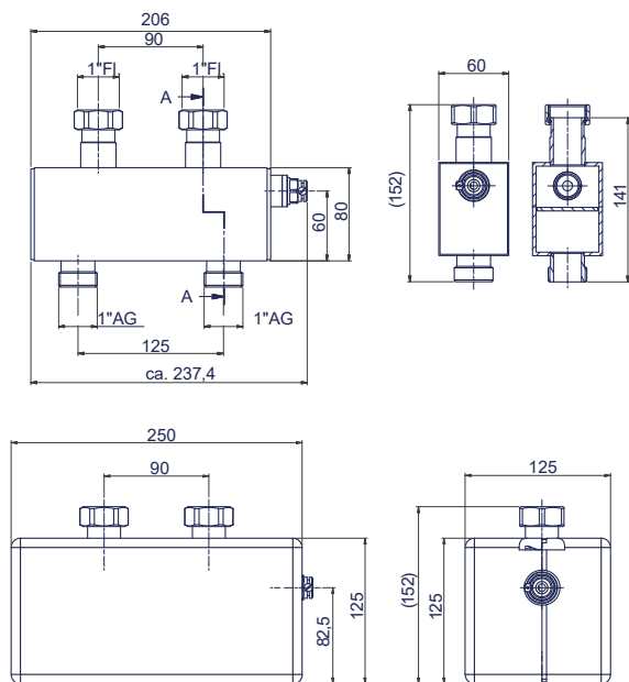
HW-Q60/80 1", 1,1 m³/h
