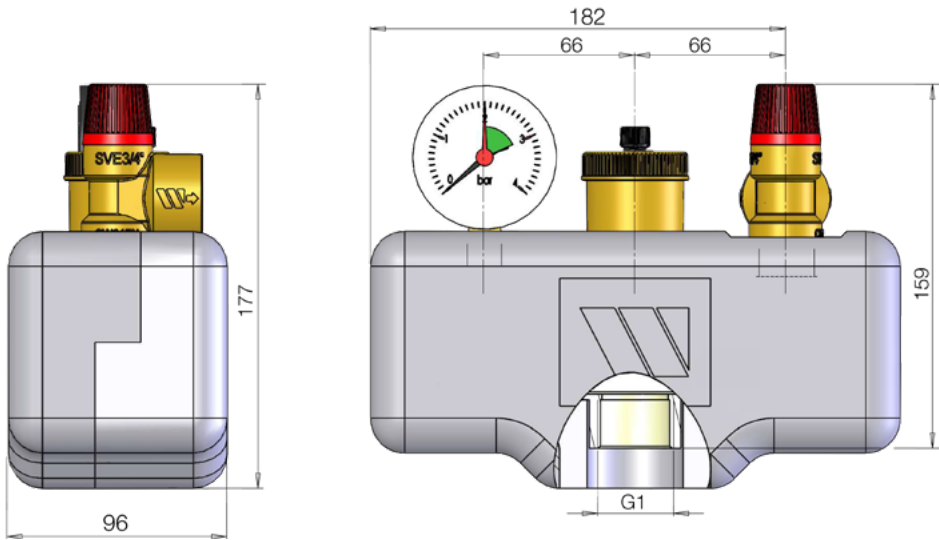
AL-ALM
